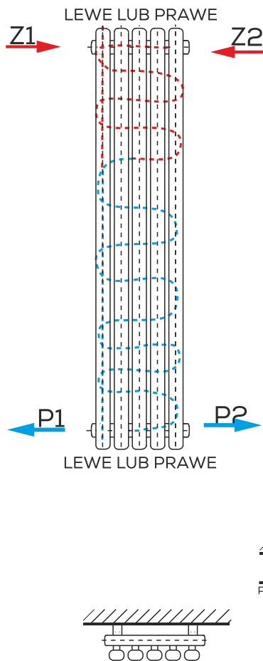
PODŁĄCZENIE STANDARDOWE GÓRA-DÓŁ
